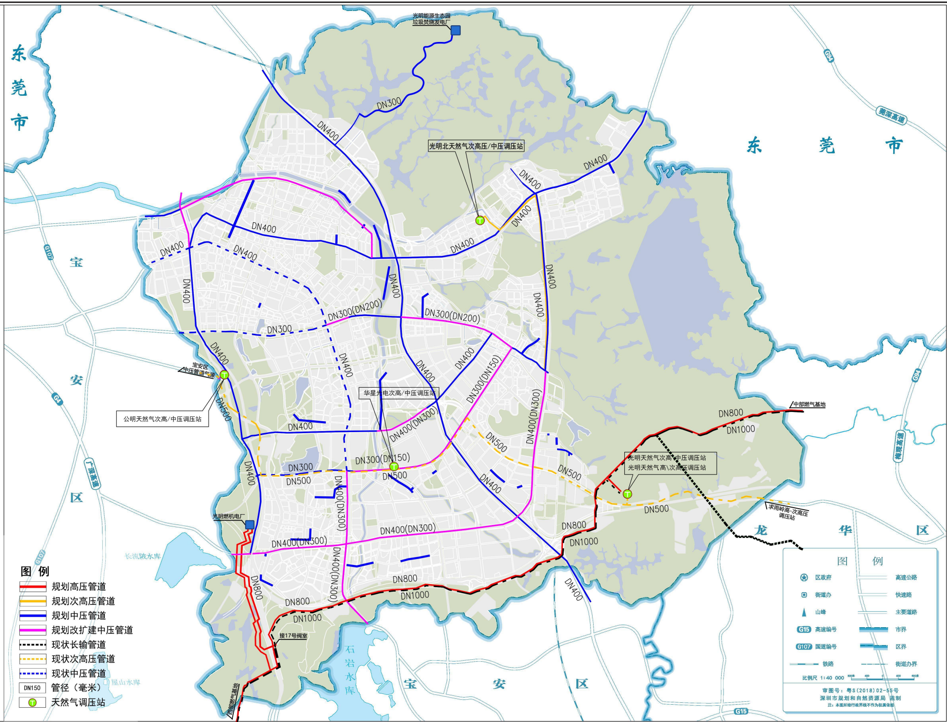
04 市政燃气管网建设规划图
