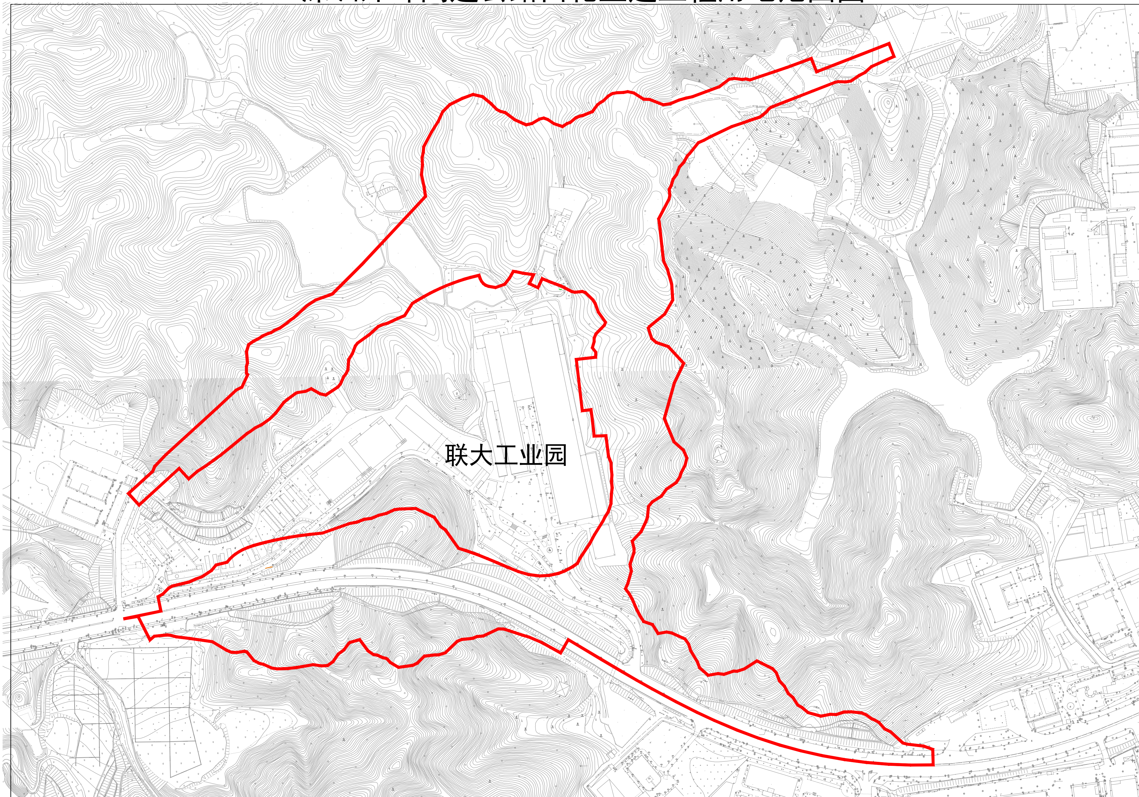
深圳外环高速公路白花互通工程用地范围图
